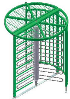
Übersteigschutz horizontal
